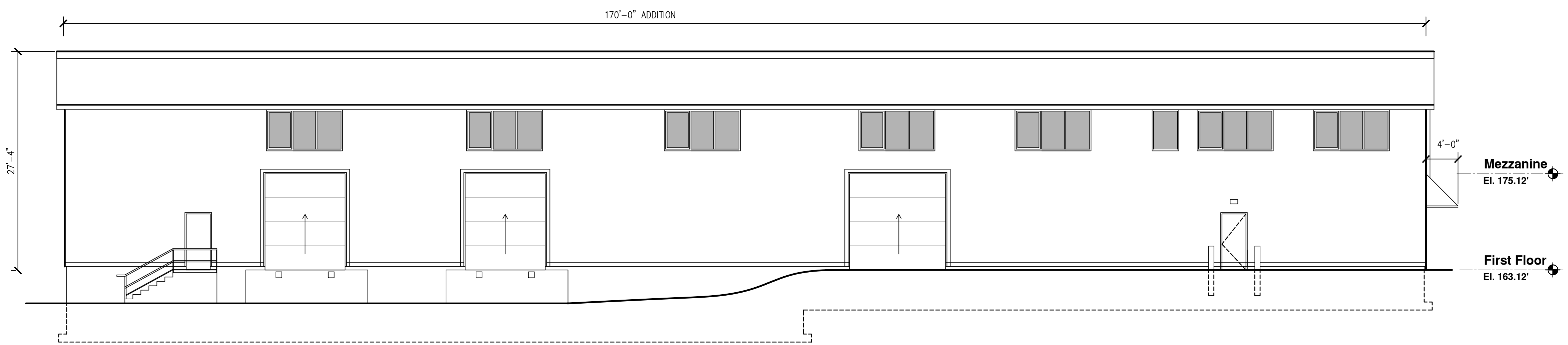
2 Elevation SCALE: 1/8" = 1'-0"
