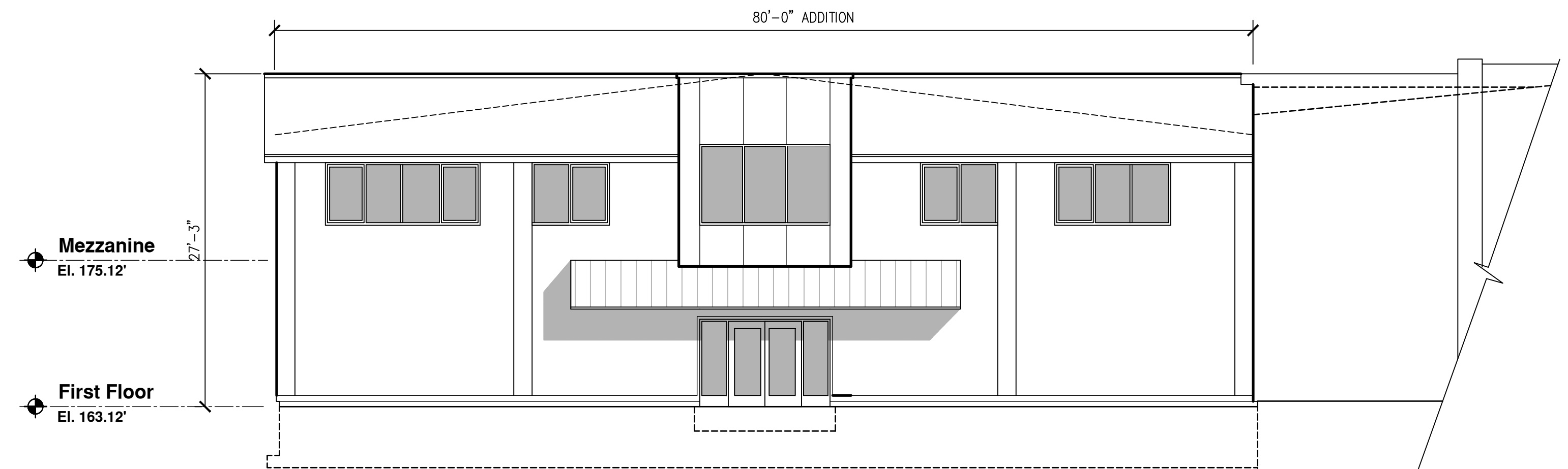
1 Elevation SCALE: 1/8" = 1'-0"
