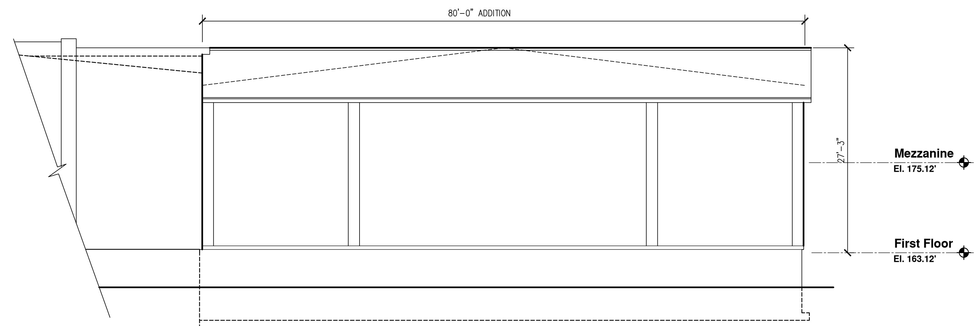
3 Elevation SCALE: 1/8" = 1'-0"
